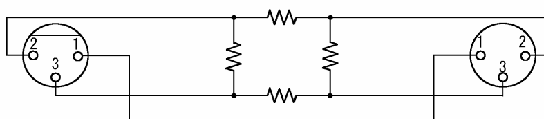
XLR-3-11Cタイプ
